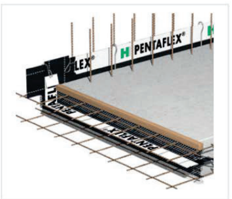
TYÖSAUMAVERKKOELEMENTTI ABS
